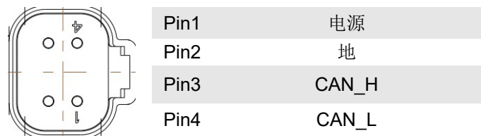
DT04-4P 四芯针式插座针脚定义
